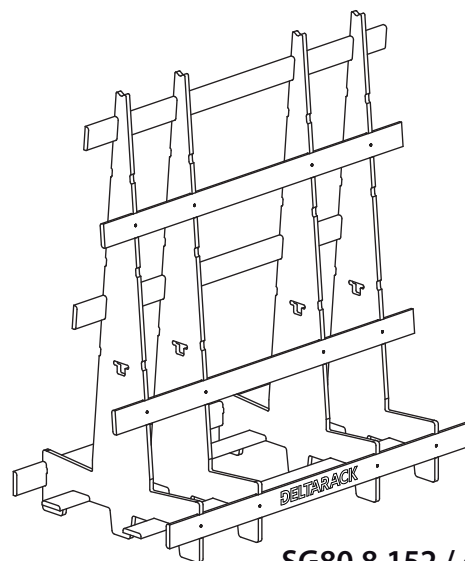
SG80.8.152 / 4 uprights
